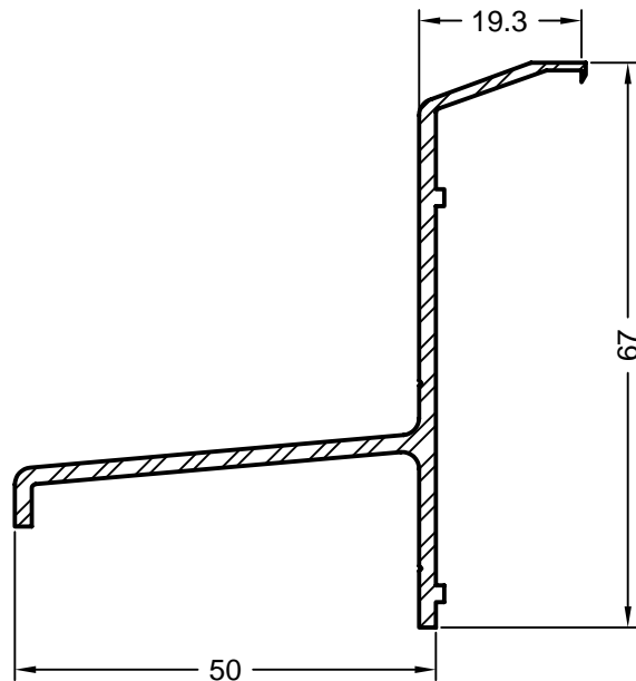
Art. 231120 natur eloxiert Verpackungseinheit: 6 m Sattelschiene Nr. 2/70 Aluminium
