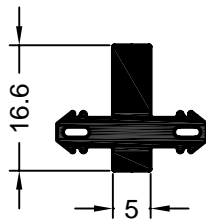
Art. 866020 grau Verpackungseinheit: 50 m Kopplungsprofil EPDM RAU-SR
