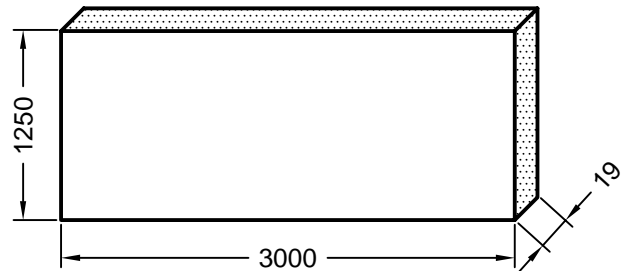
Art. 901223 Verpackungseinheit: 1 Stück 3000 x 1250 x 19 mm U = 2,1 W/m 2 K
