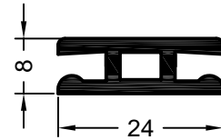
Art. 560700 01 Verpackungseinheit: 144 m Art. 593920 kaschiert Verpackungseinheit: 36 m H-Verbindungsprofil Nr. 2
