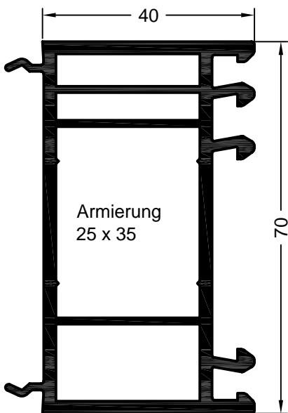
Art. 561303 01 Art. 597303 kaschiert Verpackungseinheit: 36 m Blendrahmenverbreiterung 40/70
