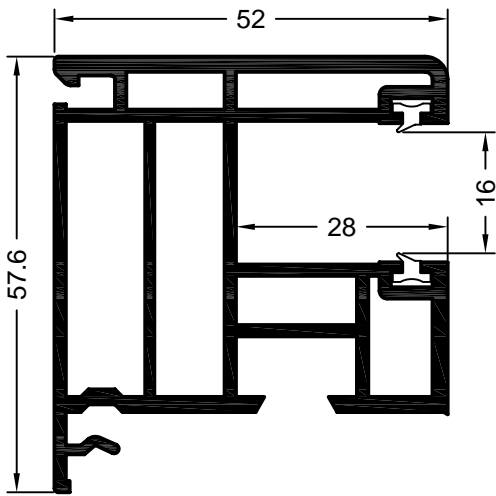
Art. 619589 05 Verpackungseinheit: 36 m Rollladenführungsschiene Nr. 2 RAU-PVC/PREN
