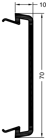
Art. 565060 01 Art. 585060 kaschiert Verpackungseinheit: 36 m Abdeckprofil 10/70
