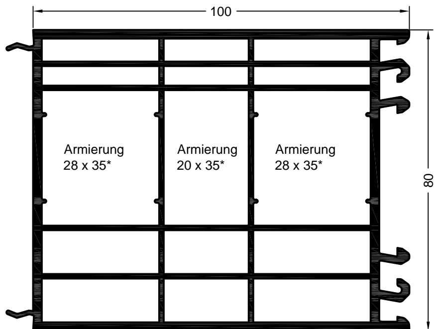
Art. 561333 01 Art. 597333 kaschiert* Verpackungseinheit: 24 m Blendrahmenverbreiterung 100/80
