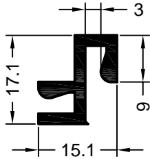
Art. 625171 01 Verpackungseinheit: 144 m Anschlussprofil
