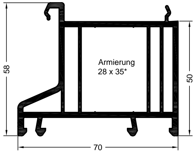
Art. 561023 01 Art. 597036 kaschiert Verpackungseinheit: 36 m Sohlbank 50/70
