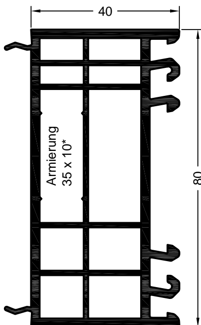
Art. 561323 01 Art. 597323 kaschiert* Verpackungseinheit: 36 m Blendrahmenverbreiterung 40/80
