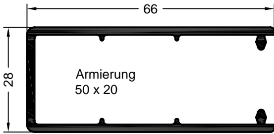
Art. 561590 01 Art. 597000 kaschiert* Verpackungseinheit: 72 m Verstärkungsprofil
