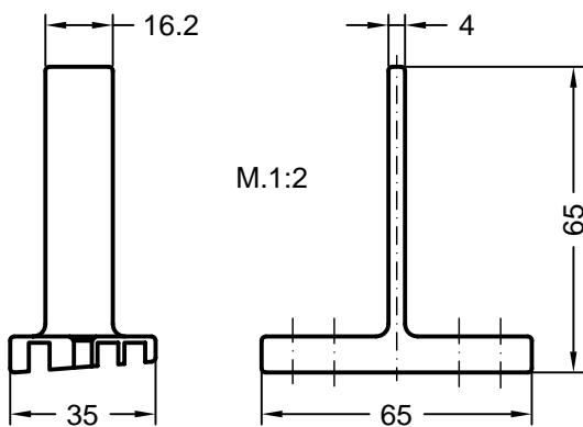
Art. 268352 Fb. beliebig Verpackungseinheit: 100 Stück Sprossenverbinder für Sprossensteg - Glasfalz RAU-PA
