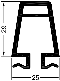
Art. 561892 01 Verpackungseinheit: 72 m Art. 597892 kaschiert Verpackungseinheit: 36 m Kopplungsprofil
