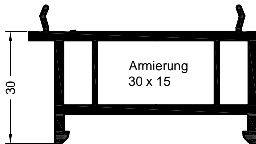
Art. 561243 01 Art. 597243 kaschiert* Verpackungseinheit: 48 m Sohlbank 30/54
