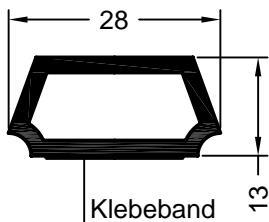
Art. 560530 01 Verpackungseinheit: 144 m Art. 593700 kaschiert Verpackungseinheit: 72 m Blindsprosse Nr. 1
