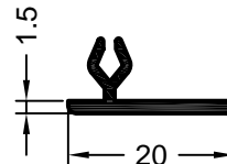
Art. 561007 Fb. beliebig, weiß* Verpackungseinheit: 144 m Füllprofil Nr. 2 für Silikonfuge (Einsatz in Verbindung mit Thermo-Design 70 nicht möglich)
