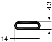
Art. 561043 Fb. beliebig Verpackungseinheit: 72 m Verbindungsfeder (Einsatz in Verbindung mit Thermo-Design 70 nicht möglich)
