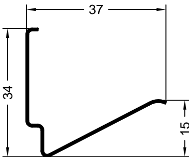
Art. 220730 Verpackungseinheit: 500 Stück Halteklammer 2/70 für Sohlbank Nr. 30 Federstahl
