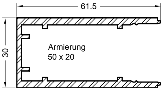
Art. 259402 weiß Verpackungseinheit: 6 m Versteifungsprofil Aluminium
