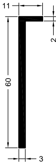
Art. 758360 01 Verpackungseinheit: 144 m Verkleidungsprofil Nr. 3
