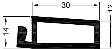
Art. 561330 01 Verpackungseinheit: 144 m Art. 597400 kaschiert* Verpackungseinheit: 36 m Verbreiterungsprofil
