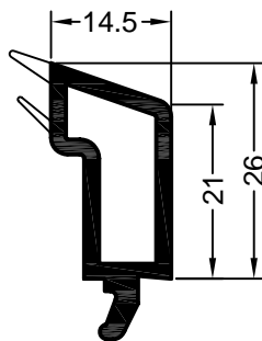
Art. 544130 01*, 05*, 15 Verpackungseinheit: 144 m Art. 574130 kaschiert* Verpackungseinheit: 72 m RAU-PVC/PREN
