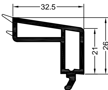
Art. 533020 01, 15 Verpackungseinheit: 144 m Art. 563020 kaschiert* Verpackungseinheit: 72 m RAU-PVC/PREN
