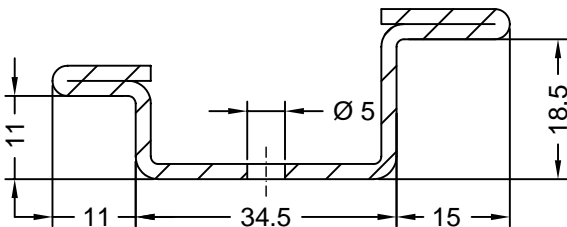
Art. 260504 Verpackungseinheit: 6 m Armierung für Rolladentraverse Nr. 1 Stahl verzinkt I_x = 8,1 \text{ cm}^4
