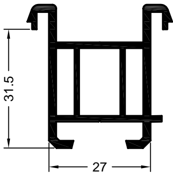
Art. 561013 01 , Fb. beliebig Art. 597035 kaschiert* Verpackungseinheit: 72 m Sohlbank Nr. 30
