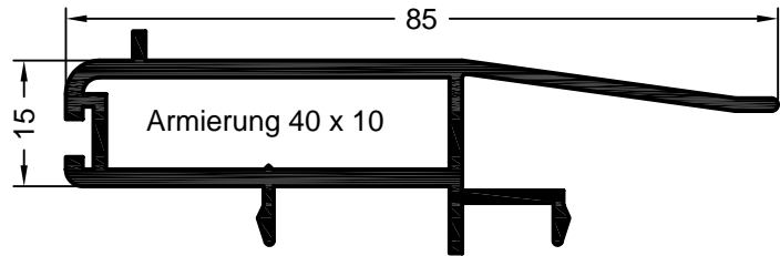
Art. 560008 01, braun Verpackungseinheit: 36 m Rolladentraverse Nr. 2
