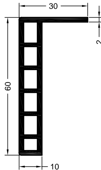
Art. 560210 01 Art. 593570 kaschiert* Verpackungseinheit: 72 m Verkleidungsprofil Nr. 4
