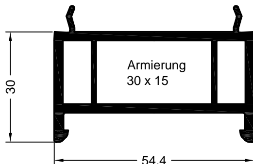
Art. 561233 01 Art. 597233 kaschiert* Verpackungseinheit: 48 m Sohlbankaufdoppelung 30/54
