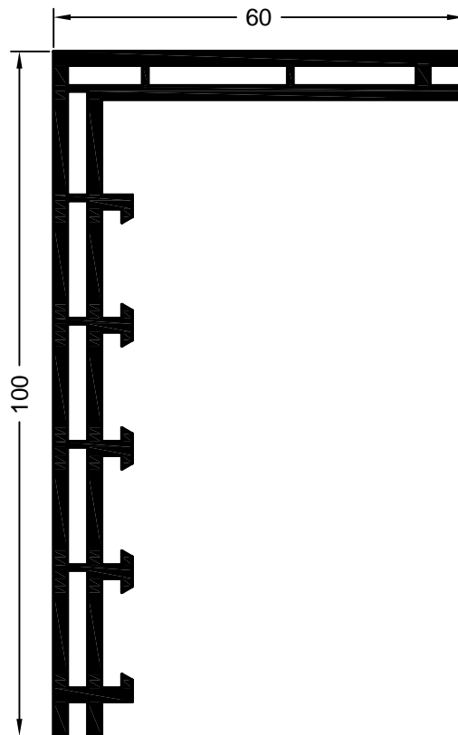
Art. 606252 01 Art. 591280 kaschiert* Verpackungseinheit: 36 m Verkleidungsprofil Nr. 1
