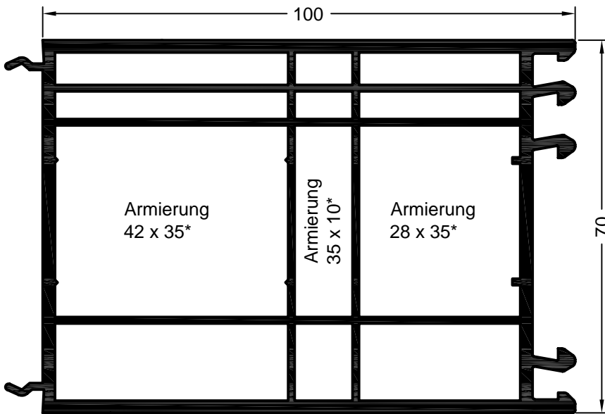
Art. 550130 01 Art. 599130 kaschiert Verpackungseinheit: 12 m Blendrahmenverbreiterung 100/70
