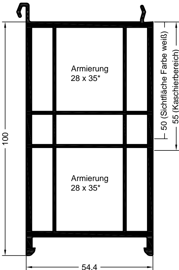
Art. 561103 01 Art. 598003 teilkaschiert* Verpackungseinheit: 24 m Sohlbank 100/54
