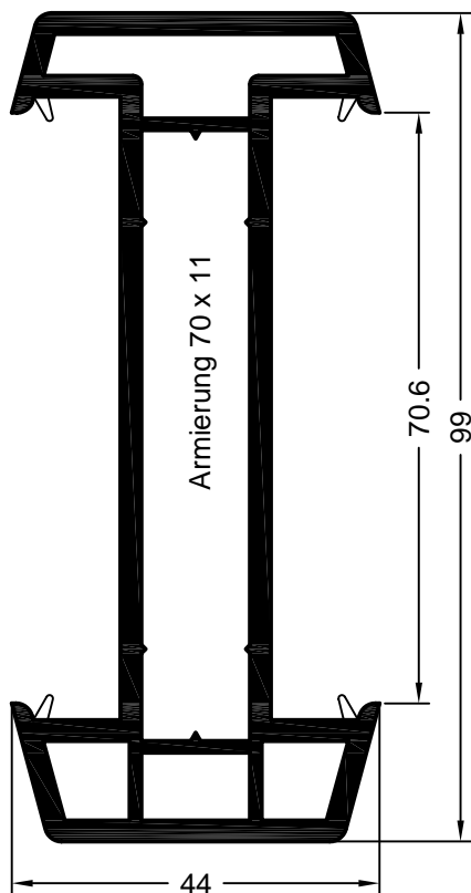
Art. 560024 01 Art. 597046 kaschiert Verpackungseinheit: 24 m Dehnstoßprofil Nr. 2/70
