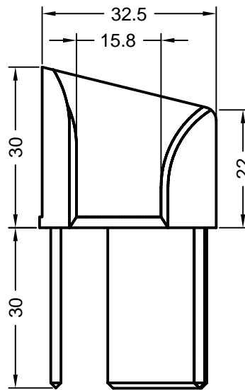
Art. 230536 rechts, weiß, braun Art. 230546 links, weiß, braun Verpackungseinheit: 100 Stück Rollladeneinlauftrichter Nr. 3 zu Führungsschiene Nr. 3 RAU-ASA
