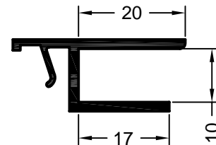
Art. 560260 01 Verpackungseinheit: 144 m Art. 591920 kaschiert Verpackungseinheit: 36 m Nutprofil Nr. 3 für Rollladenkastendeckel
