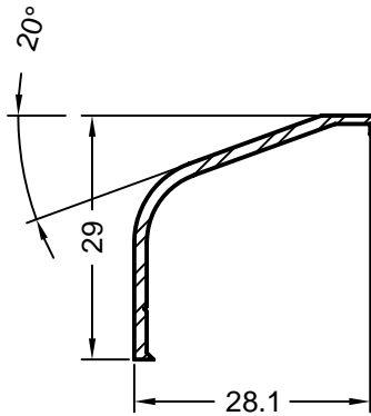
Art. 228408 natur eloxiert Verpackungseinheit: 6 m Trittschutz für Blr. 76/80 BriD Aluminium
