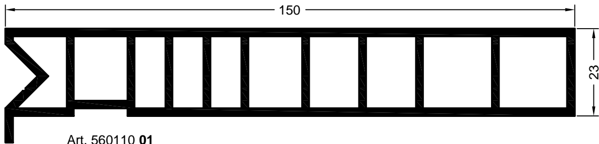
Art. 560110 01 Art. 570110 kaschiert* Verpackungseinheit: 24 m Anschlagprofil für Fallladen
