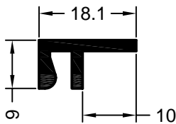
Art. 626071 01 Verpackungseinheit: 144 m Putzabzugsprofil
