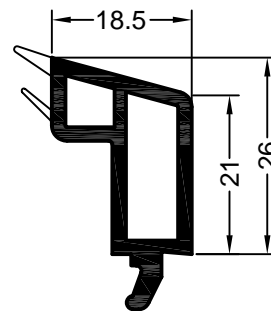
Art. 544140 01*, 05*, 15 Verpackungseinheit: 144 m Art. 574140 kaschiert* Verpackungseinheit: 72 m RAU-PVC/PREN
