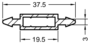
Art. 261562 Sprossensteg Verpackungseinheit: 6 m Aluminium
