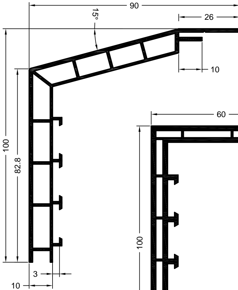
Art. 549170 01 Verpackungseinheit: 36 m Verkleidungsprofil Nr. 6
