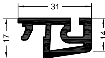
Art. 561690 01 Verpackungseinheit: 144 m Art. 596940 kaschiert* Verpackungseinheit: 72 m
