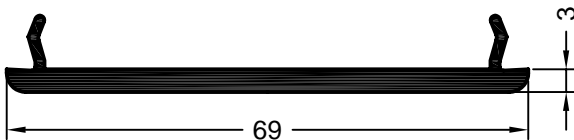
Art. 561183 weiß Verpackungseinheit: 36 m Füllprofil Nr. 1/70 für Silikonfuge
