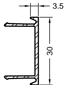
Art. 259412 weiß Verpackungseinheit: 6 m Deckkappenprofil Aluminium
