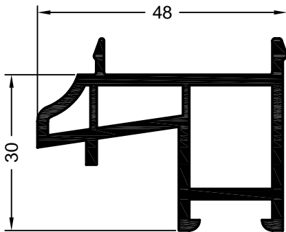
Art. 560006 01 Art. 597019 kaschiert* Verpackungseinheit: 48 m Sohlbank Nr. 42
