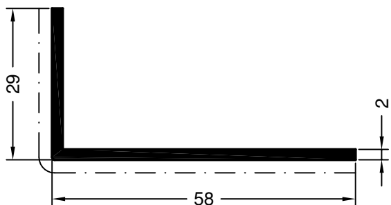
Art. 560190 01 Verpackungseinheit: 144 m Art. 591340 kaschiert Verpackungseinheit: 72 m Winkelprofil Nr. 1
