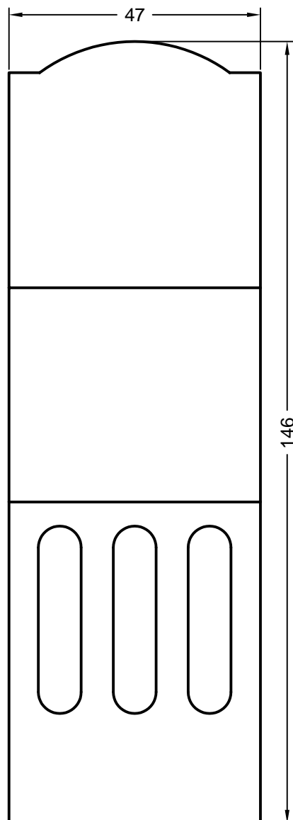
Art. 263562 weiß Verpackungseinheit: 1 Stück Zierkopf 2 für Zierprofil Nr. 2 RAU-ASA
