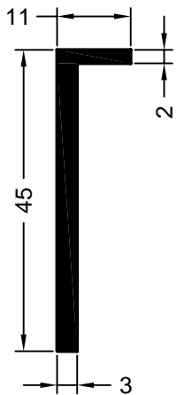
Art. 758370 01 Verpackungseinheit: 144 m Verkleidungsprofil Nr. 2
