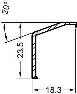
Art. 248786 natur eloxiert Verpackungseinheit: 6 m Trittschutz Nr. 2 Aluminium
