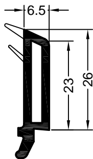
Art. 544110 01*, 05*, 15* Verpackungseinheit: 144 m Art. 574110 kaschiert* Verpackungseinheit: 72 m RAU-PVC/PREN
