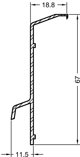
Art. 222700 natur eloxiert Verpackungseinheit: 6 m Sattelschiene Nr. 1/70 Aluminium
