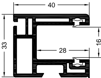
Art. 625533 05 Verpackungseinheit: 72 m Art. 625543 kaschiert* Verpackungseinheit: 24 m Rollladenführungsschiene Nr. 3 RAU-PVC/PREN
