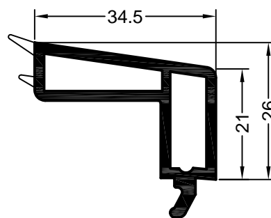
Art. 533030 01, 15 Verpackungseinheit: 144 m Art. 563030 kaschiert* Verpackungseinheit: 72 m RAU-PVC/PREN
