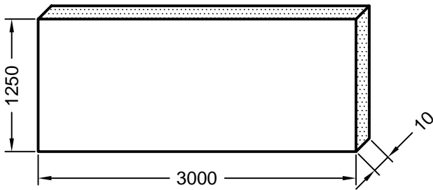
Art. 901243 Verpackungseinheit: 2 Stück 3000 x 1250 x 10 mm U = 3,0 W/m 2 K
