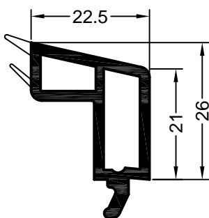
Art. 545001 01, 15 Art. 565001 kaschiert* Verpackungseinheit: 144 m RAU-PVC/PREN
