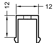
Art. 258690 Verpackungseinheit: 100 Stück Klemmstück Aluminium
