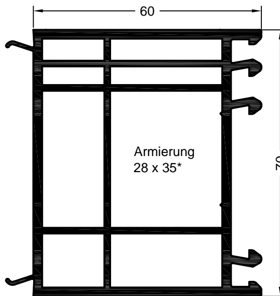
Art. 561113 01 Art. 597113 kaschiert* Verpackungseinheit: 36 m Blendrahmenverbreiterung 60/70
