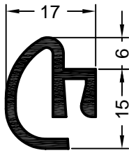
Art. 561700 01, braun Verpackungseinheit: 144 m Rolladentraverse Nr. 1
