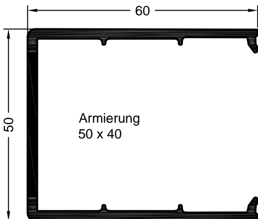
Art. 259402 weiß Verpackungseinheit: 6 m Versteifungsprofil Aluminium
