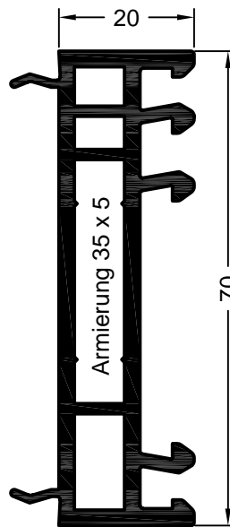
Art. 561293 01 Art. 597293 kaschiert Verpackungseinheit: 36 m Blendrahmenverbreiterung 20/70
