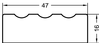
Art. 257833 weiß Verpackungseinheit: 100 Stück Endkappe für Zierprofil Nr. 1 RAU-ASA
