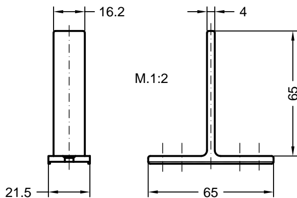
Art. 268362 Fb. beliebig Verpackungseinheit: 100 Stück Sprossenverbinder für Sprossensteg - Kreuzstoß RAU-PA
