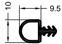
Art. 865520 schwarz Verpackungseinheit: 200 m Dichtung für Dehnstoßprofil Nr. 2/70 RAU-SR
