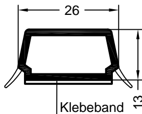
Art. 265506 01, 15 Art. 597506 kaschiert Verpackungseinheit: 60 m Blindsprosse 26 RAU-PVC/PREN
