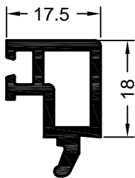
Art. 575054 01* Verpackungseinheit: 144 m
