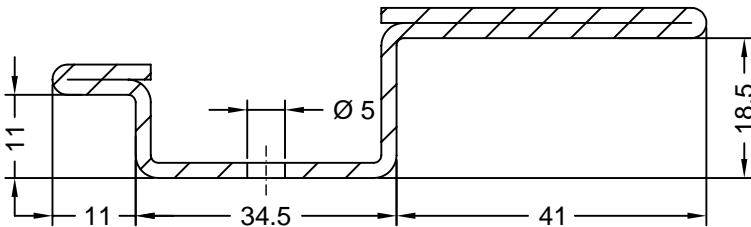
Art. 269231 Armierung für Rolladentraverse Nr. 1 Verpackungseinheit: 6 m Stahl verzinkt I_x = 21 \text{ cm}^4
