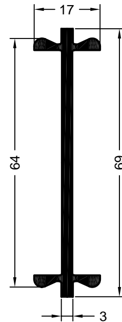
Art. 546301 01 Verpackungseinheit: 72 m Verbindungsprofil 3/70
