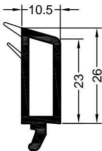
Art. 544120 01*, 05*, 15* Verpackungseinheit: 144 m Art. 574120 kaschiert* Verpackungseinheit: 72 m RAU-PVC/PREN
