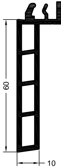
Art. 561910 01 Art. 597690 kaschiert* Verpackungseinheit: 36 m Sohlbank Nr. 31/60
