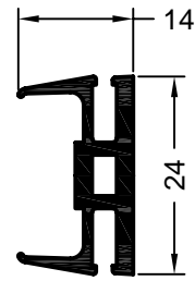
Art. 561600 01 Verpackungseinheit: 72 m Halteprofil
