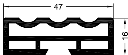
Art. 257853 01 Art. 597012 kaschiert* Verpackungseinheit: 72 m Zierprofil Nr. 1
