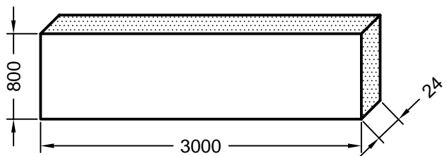
Art. 901233 Verpackungseinheit: 1 Stück 3000 x 800 x 24 mm U = 1,8 W/m 2 K
