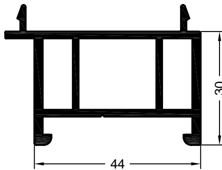
Art. 561740 01 Verpackungseinheit: 72 m Art. 596980 kaschiert* Verpackungseinheit: 36 m Sohlbank Nr. 33
