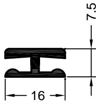
Art. 732460 01 Verpackungseinheit: 144 m Art. 590010 kaschiert Verpackungseinheit: 36 m H-Verbindungsprofil Nr. 1
