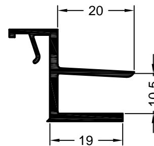
Art. 626051 01 Verpackungseinheit: 144 m Nutprofil Nr. 1 für Rollladenkastendeckel
