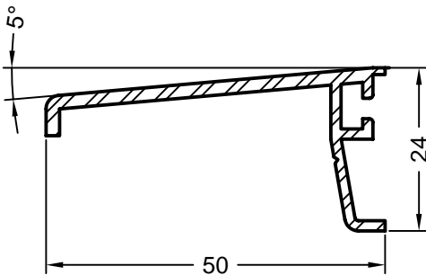
Art. 248786 natur eloxiert Verpackungseinheit: 6 m Trittschutz Nr. 2 Aluminium
