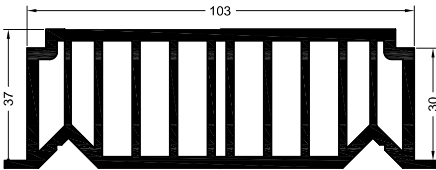
Art. 560110 01 Art. 570110 kaschiert* Verpackungseinheit: 24 m Anschlagprofil für Fallladen
