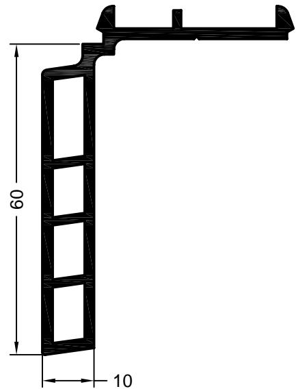
Art. 561710 01 Art. 596970 kaschiert Verpackungseinheit: 48 m Sohlbank Nr. 32
