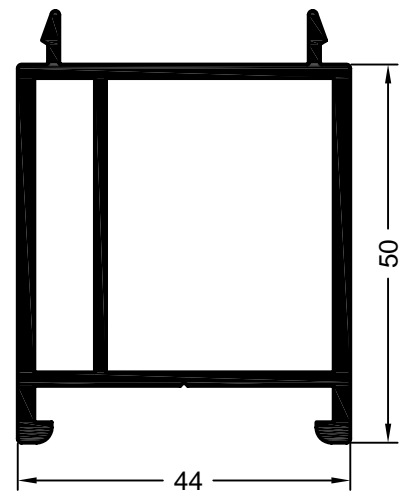
Art. 561790 01 , Fb. beliebig Verpackungseinheit: 36 m Sohlbank Nr. 34
