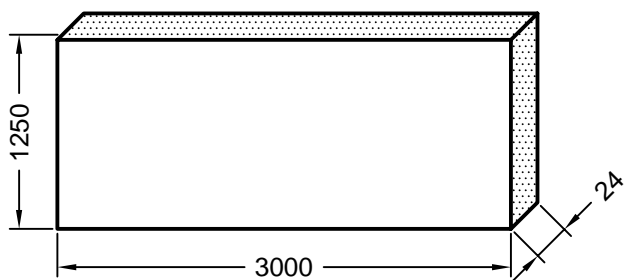
Art. 901683* Verpackungseinheit: 1 Stück 3000 x 1250 x 24 mm U = 1,8 W/m 2 K
