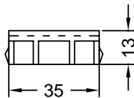
Art. 246691 Fb. beliebig Verpackungseinheit: 100 Stück Distanzklotz 13 für Dehnstoßprofil Nr. 2/70 (M 1:2) RAU-PS
