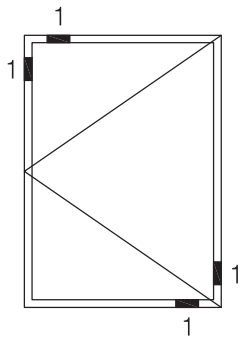
Abb. 5: Drehflügel
