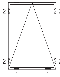
Abb. 7: Kippflügel
