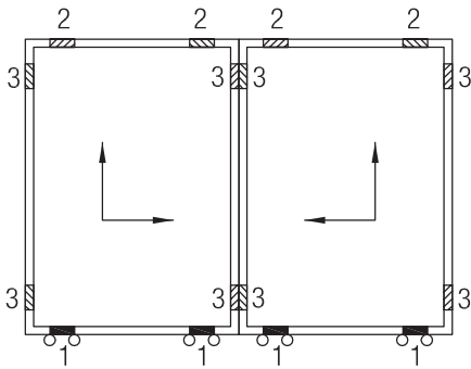
Abb. 10: Horizontal-Schiebe-Element mit je 2 Laufwägen pro Flügel
