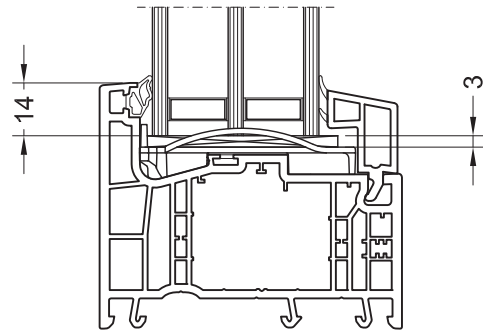
Abb. 3: Blendrahmen
