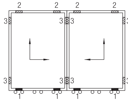
Abb. 11: Horizontal-Schiebe-Element mit je 3 Laufwägen pro Flügel
