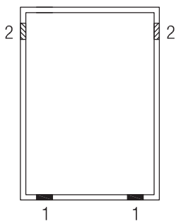
Abb. 8: Festverglasung: Glasgewicht ≤ 200 kg
