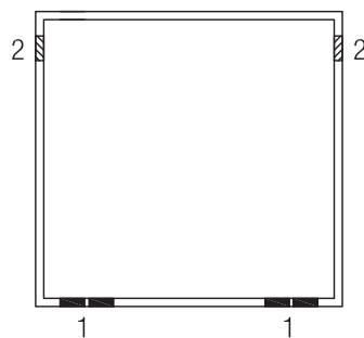
Abb. 9: Festverglasung: Glasgewicht > 200 kg bis 400 kg
