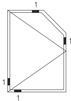
Abb. 13: 5-Eck Schrägfenster Dreh
