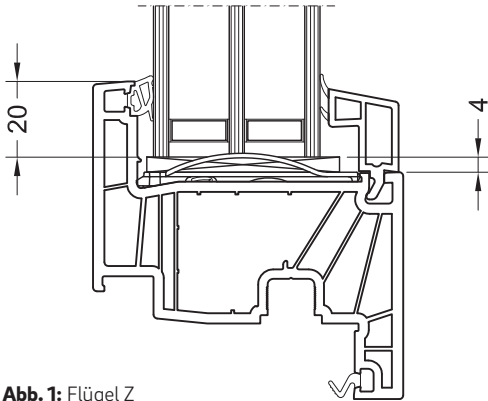
Abb. 1: Flügel Z
