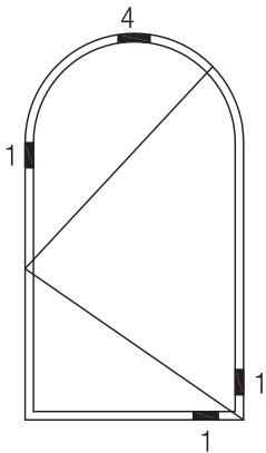
Abb. 12: Bogenfenster Dreh
