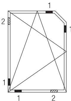
Abb. 16: 5-Eck Schrägfenster Dreh-Kipp
