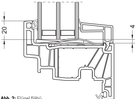
Abb. 2: Flügel fläbü
