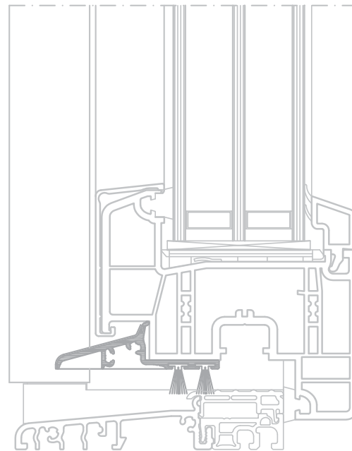
Wetterschenkel Fenstertür
