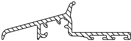
ALU TOP Wetterschenkel
