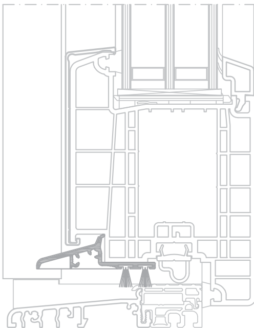
Wetterschenkel Haustür
