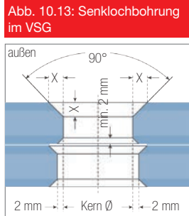
Abb. 10.13: Senklochbohrung im VSG
