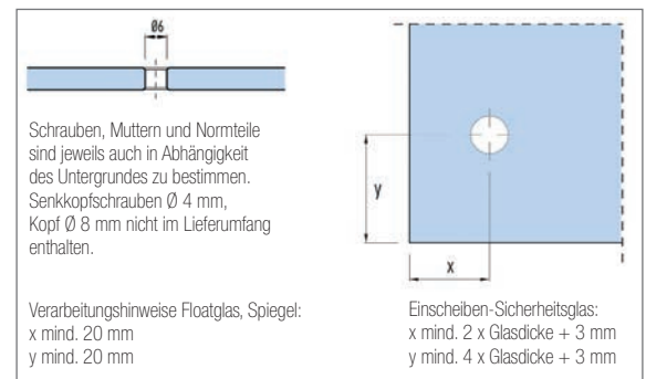
Abb. 8.20: Technischer Aufbau
