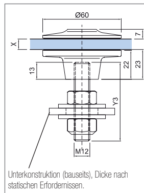
Abb. 8.24: Systemschnitt
