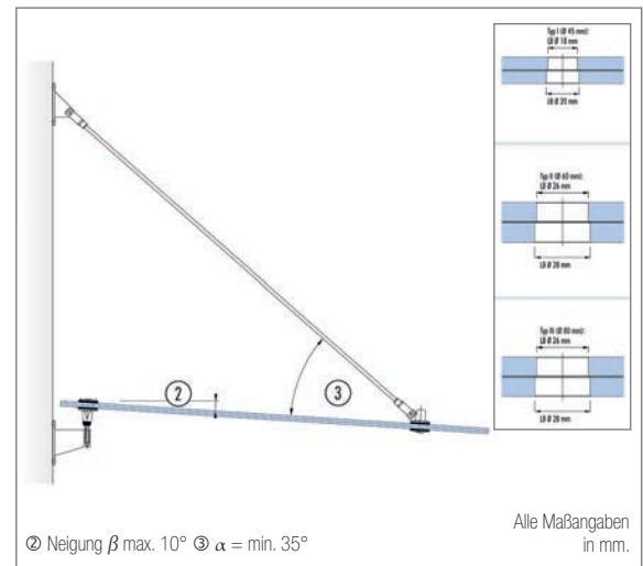
Abb. 8.10: Montageansicht / Glasbohrung
