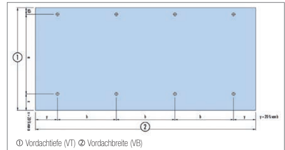
Abb. 8.10: Montageansicht / Glasbohrung
