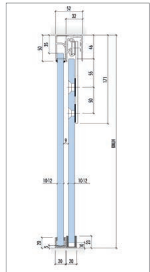
Abb. 8.44: Systemschnitt
