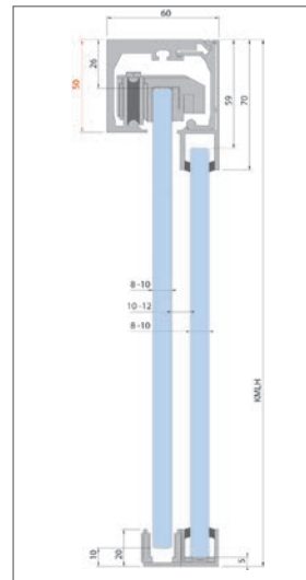
Abb. 8.39: Taschenmontage
