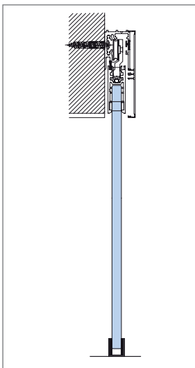
Abb. 8.42: Typ C
