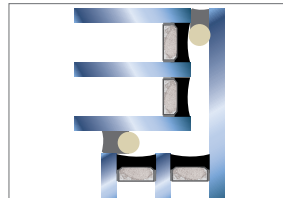
Abb. 3.10: Variante 1 d: Ecke (3-fach IG) (Prinzipdarstellung) [1]
