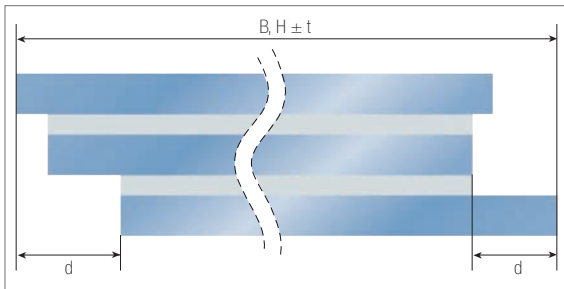
Abb. 10.15: Versatz
