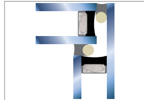
Abb. 3.8: Variante 1 c: Ecke (2-fach IG) (Prinzipdarstellung) [1]
