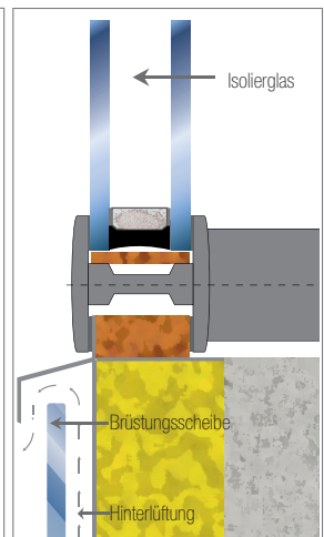
Abb. 6.13: Kaltfassade (Systemschnitt)
