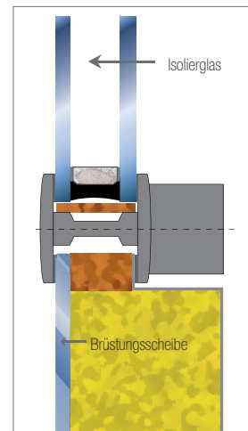
Abb. 6.12: Warmfassade (Systemschnitt)
