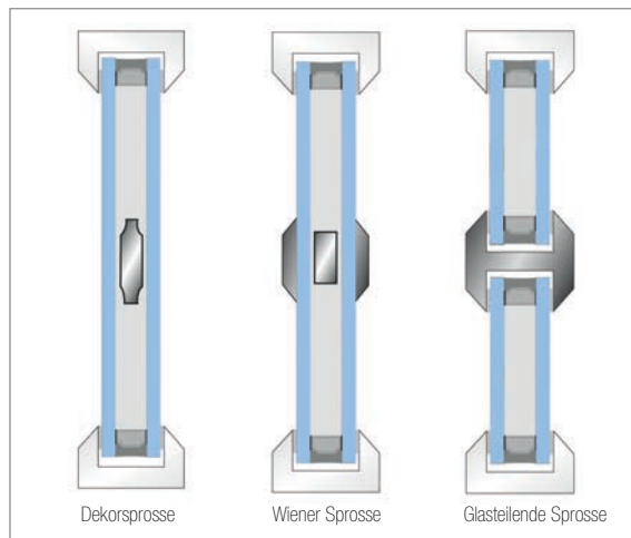
Abb. 10.36: Sprossenarten
