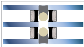
Abb. 3.6: Variante 1 b: Stoßfuge (3-fach IG) (Prinzipdarstellung) [1]
