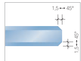
Abb. 10.5: Kantenbearbeitung
