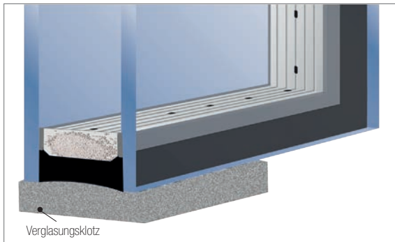
Abb. 10.40: Klotzungstechnik
