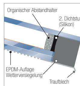
Abb. 10.25: Fehlerhafte Traufpunktversiegelung
