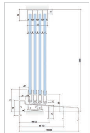
Abb. 8.54: Systemschnitt
