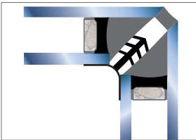
Abb. 3.16: Variante 2 c: Ecke (2-fach IG) (Prinzipdarstellung) [1]
