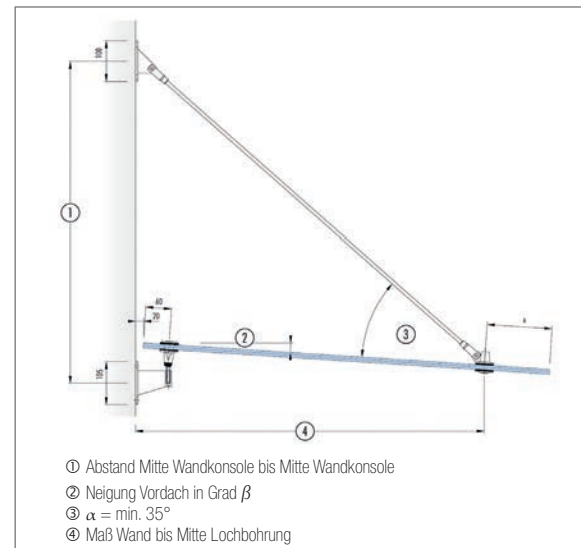
Abb. 8.6: Montageansicht
