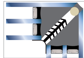
Abb. 3.18: Variante 2 d: Ecke (3-fach IG) (Prinzipdarstellung) [1]
