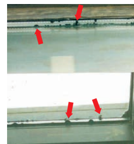
Abb. 10.24 Auflösen der Butyl-Dichtung durch Migration
