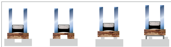
Abb. 10.17: Mögliche Klotzungen
