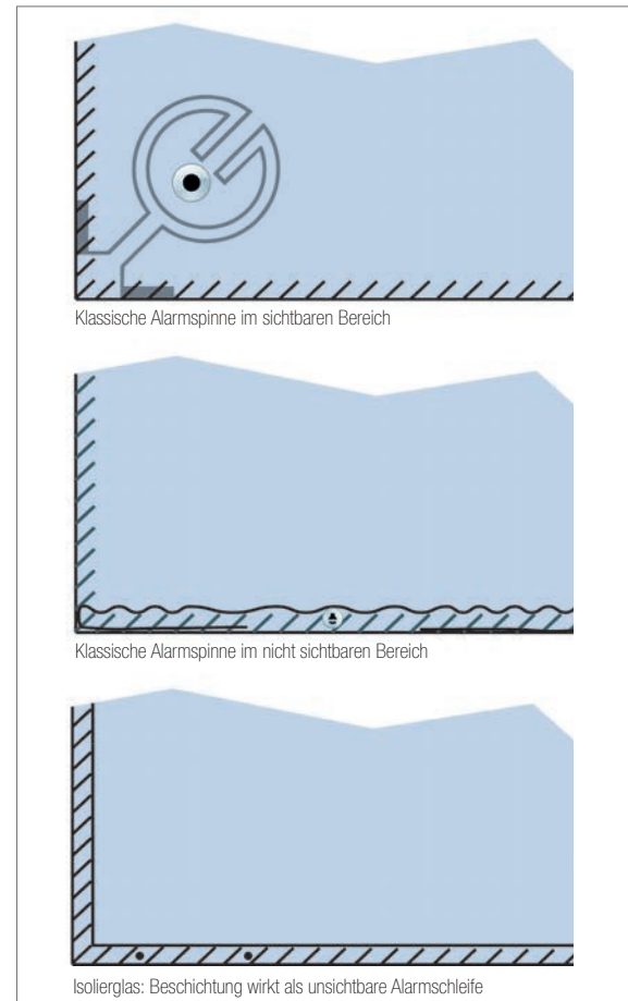
Abb. 2.10: Varianten der Leiterschleifen (Spinne)
