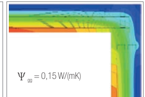
Abb. 3.11: Isothermendarstellung [1]
