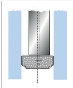
Abb. 10.38: Parallelität
