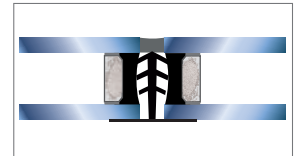
Abb. 3.12: Variante 2 a: Stoßfuge (2-fach IG) (Prinzipdarstellung) [1]
