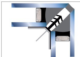
Abb. 3.24: Variante 3 c: Ecke (2-fach IG) (Prinzipdarstellung) [1]
