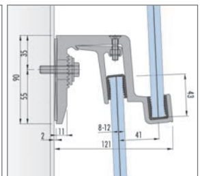
Abb. 8.32: Systemschnitt Mitte
