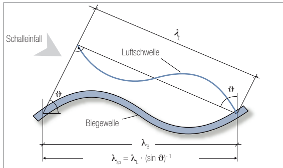
Abb. 5.3: Koinzidenzfrequenz
