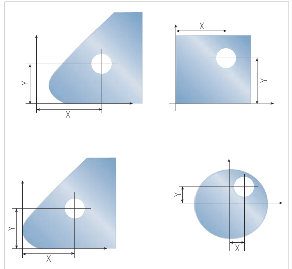
Abb. 10.10: Lochlage
