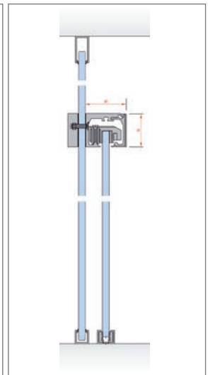
Abb. 8.38: Systemschnitt
