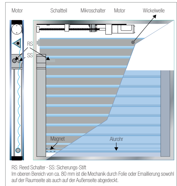
Abb. 6.10: UNIGLAS® | SHADE Folien-System Gesamtansicht raumseitig
