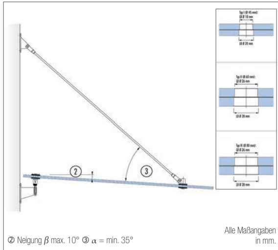
Abb. 8.8: Montageansicht / Glasbohrung
