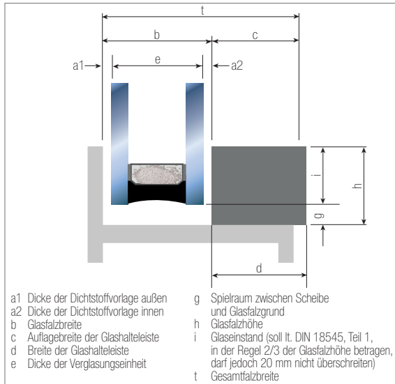
Abb. 10.16: Falzabmessungen
