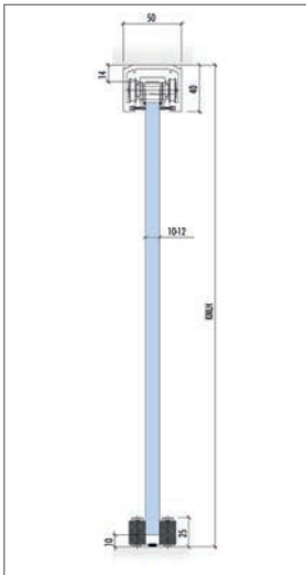
Abb. 8.45: Systemschnitt
