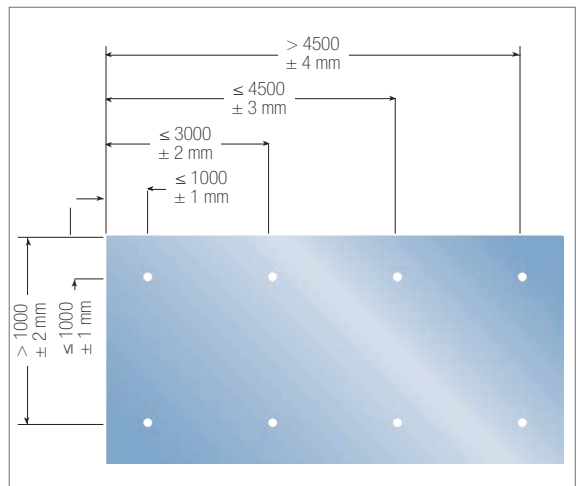
Abb. 10.11: Lochbohrungslagen
