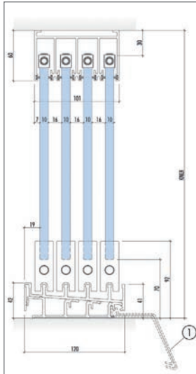
Abb. 8.55: Systemschnitt
