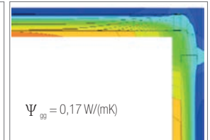
Abb. 3.9: Isothermendarstellung [1]
