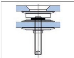
Abb. 8.4: Systemschnitt
