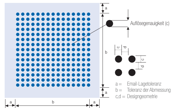
Abb. 2.7: Lage- und Designtoleranzen der Abmessung bei bedruckten Gläsern
