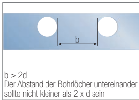
Abb. 10.8: Lage benachbarter Bohrlöcher
