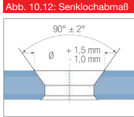
Abb. 10.12: Senklochabmaß
