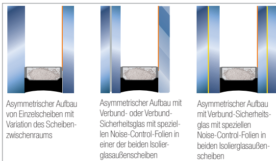
Abb. 5.5: UNIGLAS® | PHON: 3 Kategorien Schallschutz-Isoliergläser
