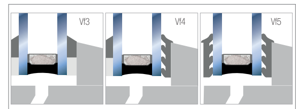
Abb. 10.19: Verglasungssysteme
