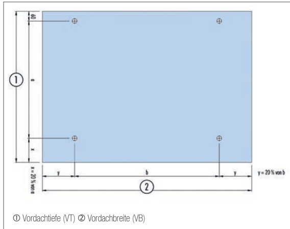
Abb. 8.7: Bohrlochvorlage
