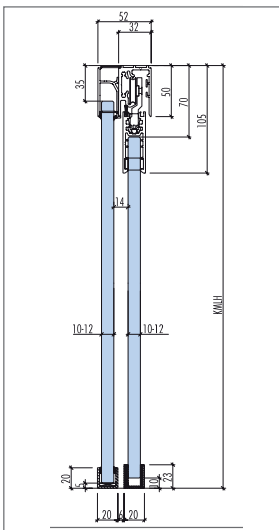
Abb. 8.43: Typ D
