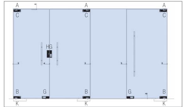
Abb. 8.58: Beispiel Ganzglasanlage mit Oberlicht
