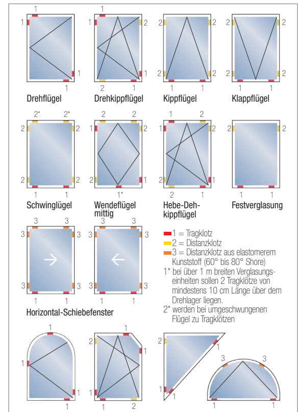
Abb. 10.18: Klotzungsvorschläge Auszug aus „Technische Richtlinie des Glaserhandwerks Nr. 3, Ausgabe 1997“
