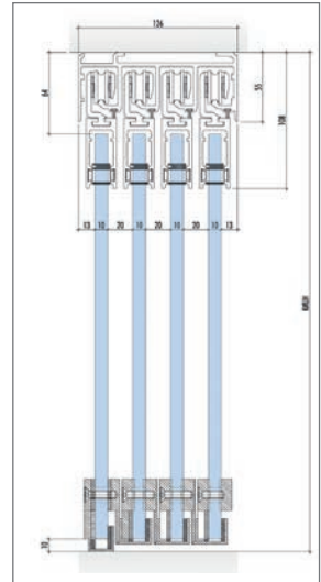
Abb. 8.47: Systemschnitt
