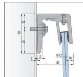
Abb. 8.31: Systemschnitt oben
