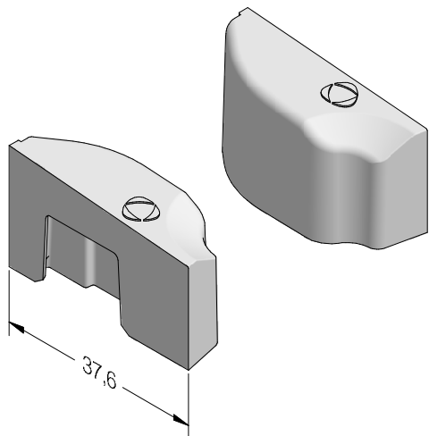
Set Windstopp AD SYNEGO®
