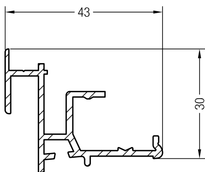
Ausgleichsprofil SYNEGO®
