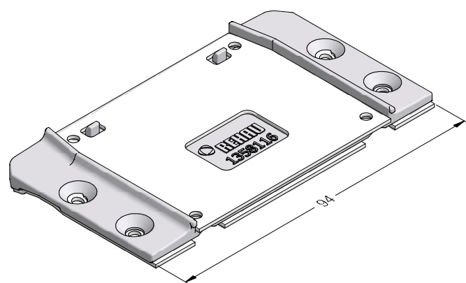
Mechanischer Verbinder Pfosten 124 AD SYNEGO®
